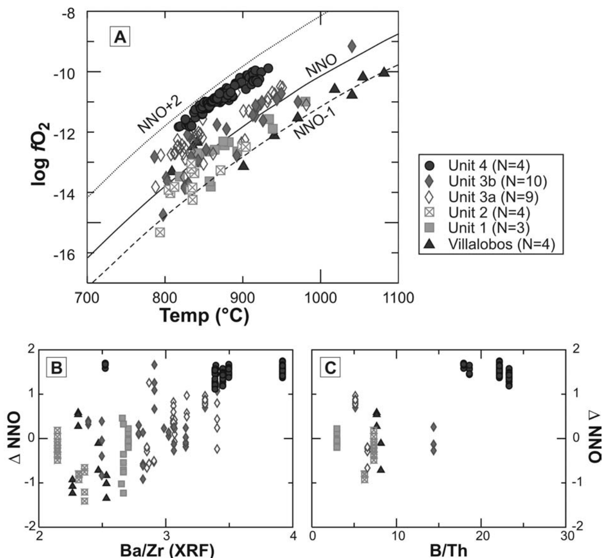
Figure 4 : Variation des conditions de température et de fugacité d'oxygène des magmas dans la zone d'étude (A). L'augmentation progressive de l'état d'oxydation des magmas est accompagnée par une augmentation des rapports d'éléments en trace caractéristiques de la participation de fluides.
