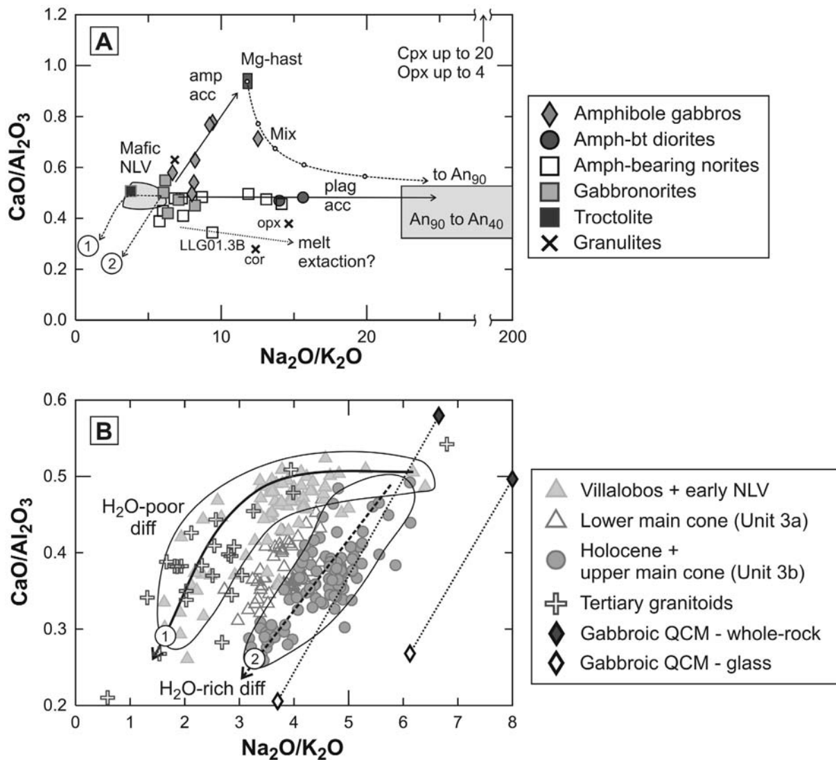
Figure 5 : En haut, compositions des xénolites du VNL. On peut y distinguer les tendances d'accumulation d'amphibole et de plagioclase. La différenciation de magmas basaltiques (zone grise) par l'extraction de plagioclase produit le trend 1, tandis que la stabilisation d'amphibole produit le trend 2. En bas, le trend de différenciation des magmas dans des conditions de faible teneur en eau est représenté par les unités anciennes du VNL. Les unités récentes suivent un trend dominé par le fractionnement d'amphibole produisant des magmas évolués avec Na_2O/K_2O élevés. L'unité 3a suit un trend intermédiaire.
