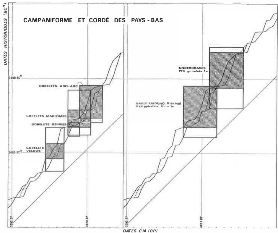
Fig. 11. Calibration de la séquence Cordé-Campaniforme aux Pays-Bas d'après la courbe de la Jolla (Suess 1979). (Datations de base d'après Lan-ting et van der Waals 1976).
