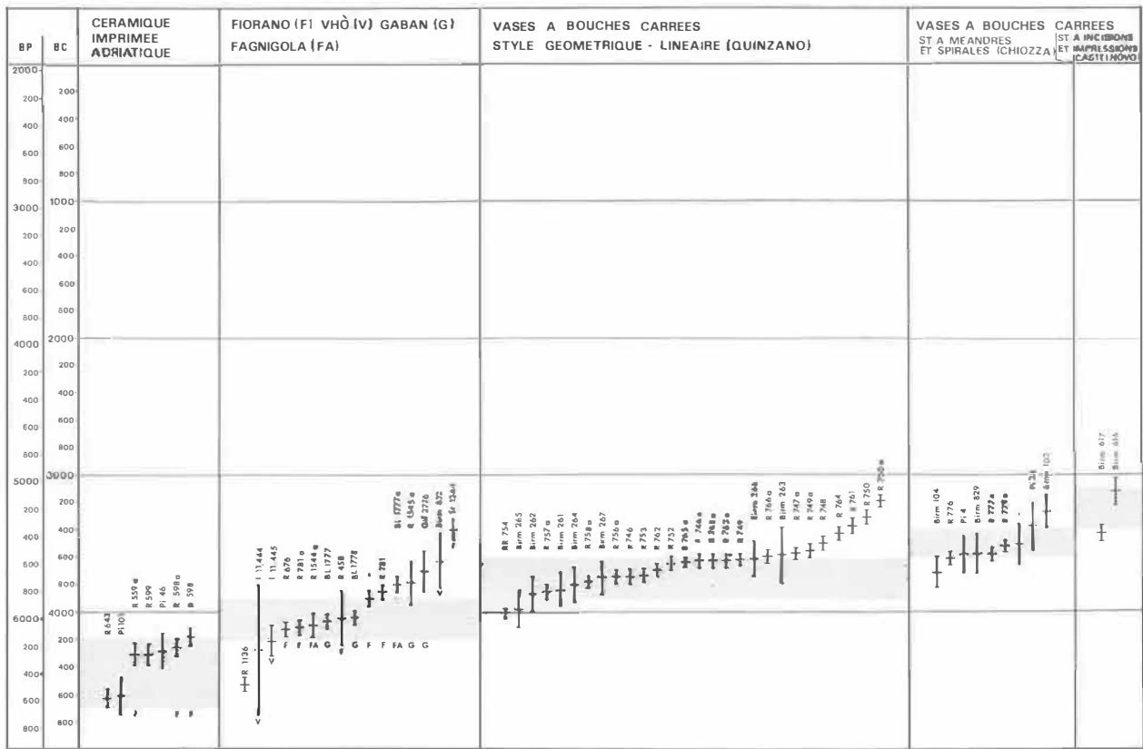
Fig. 8. Datations 14 C conventionnelles (BP/BC) de l'Italie septentrionale et extension probable des ensembles culturels, Bassin du Pô: Céramique imprimée adriatique, Néolithique ancien tardif et vases à Bouches carrées.
