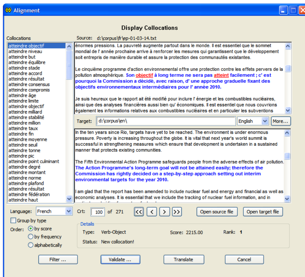
Figure 1. L'interface du concordancier bilingue pour les collocations
