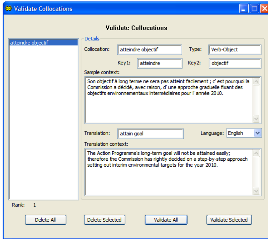
Figure 2. L'interface du module de validation de collocations
