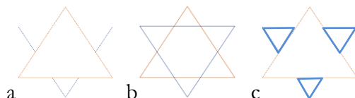
Fig. 8 : Trois manières possibles de percevoir les deux triangles à partir de la production de M. dans la figure 6
