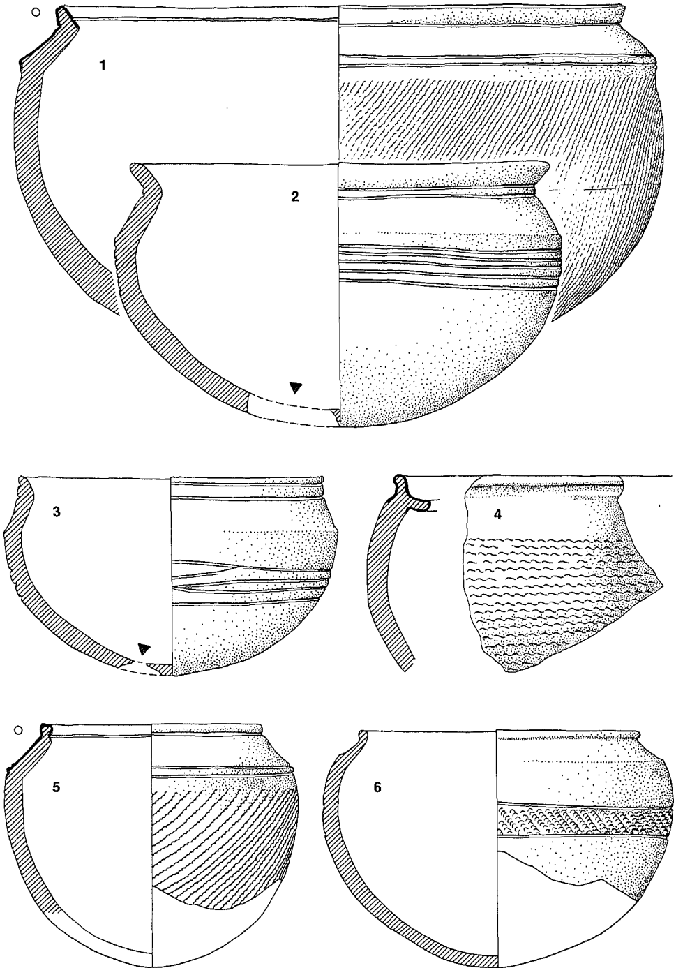
FIG. 11.— Sine-Ngayène. Fouilles G. Thilmans et C. Descamps 1975-76 (sauf 4?). Céramique de cercles 25 (3 et 6), 28 (1, 2 et 5) et 31 (4). Signes diacritiques, voir fig. 6. Triangles: fonds perforés intentionnellement. Ech. 1:2. (Dessin G. Pignat). Collection IFAN (Dakar).
