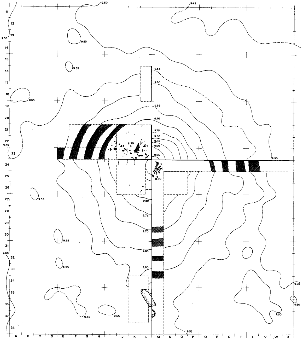
FIG. 2.—Santhiou Kohel, Mbolo Tobé. Plan général du tumulus 43. Position des sondages et emplacement des sépultures centrales. Equidistance 5 cm, carroyage métrique. (Dessin Y. Reymond).
