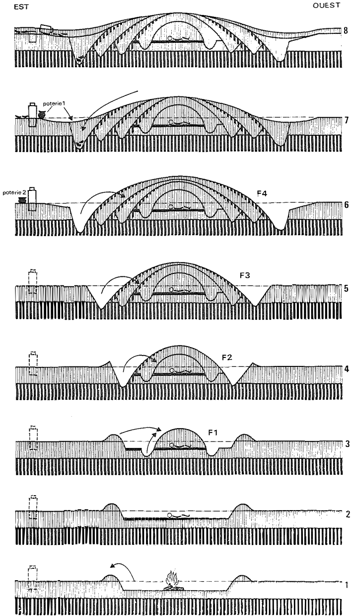
FIG. 8.—Santhiou Kohel Mbolop Tobé. Tumulus 43. Les diverses phases de la construction du tumulus. Critique de la phase I, voir texte. (Dessin S. Aeschlimann).
