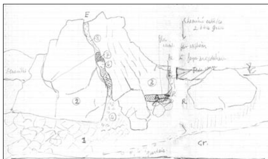
Fig. 6 Vue latérale de la fissure aux squelettes, avec insertion de l'abri Jayet à l'ouest et blocs de l'abri. Croquis d'Adrien Jayet daté du 13.12.1947 (carnet 9).
