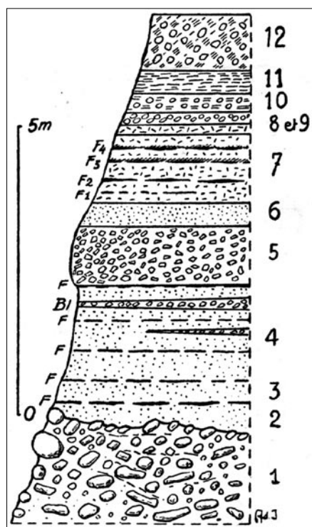
Fig. 11 Coupe de référence de la gravière Achard, montrant la succession des limons jaunes, publiée par Adrien Jayet en 1946.
